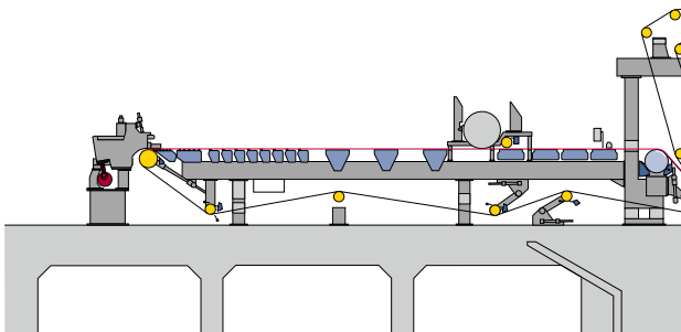
Fourdrinier machine
