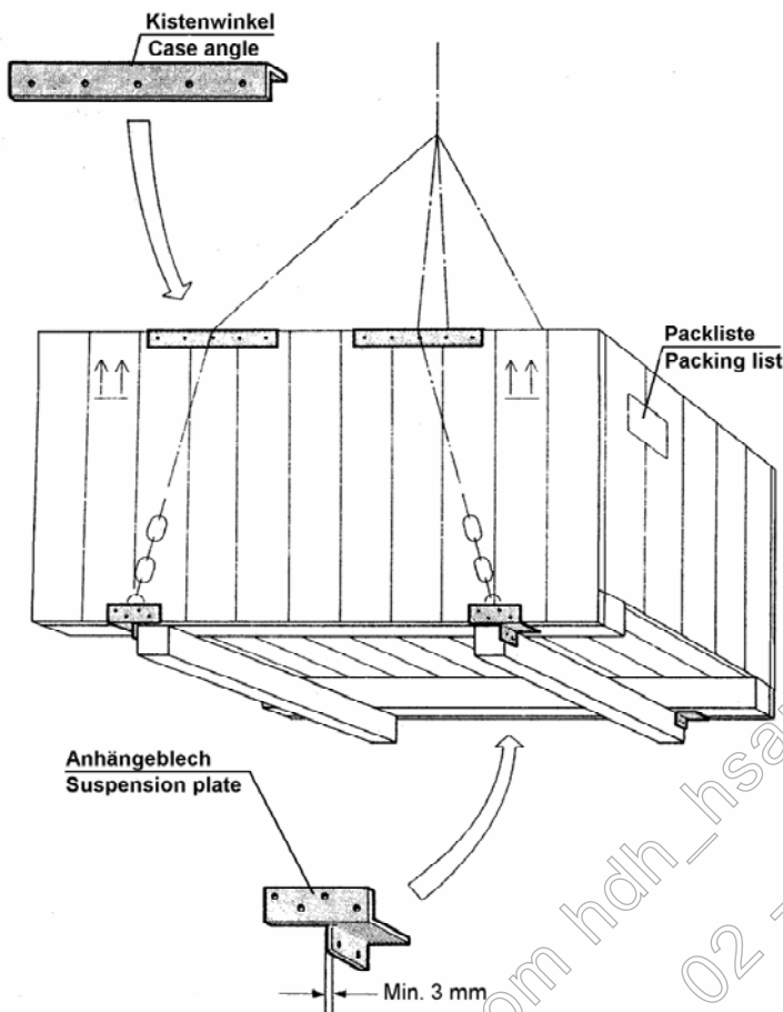
Abbildung 17: Anbringen von Schwergutbeschlagen
